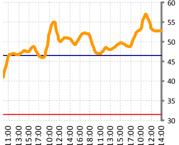
Relative Strength In (14), посл. 4 дня
