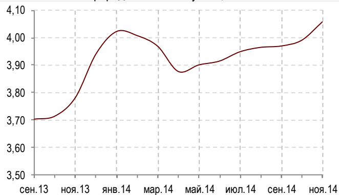
Природный газ Henry Hub, NYMEX
