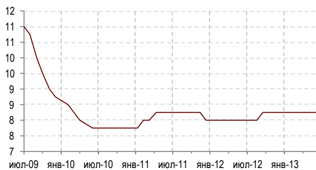
Ставка рефинансирования ЦБ РФ
