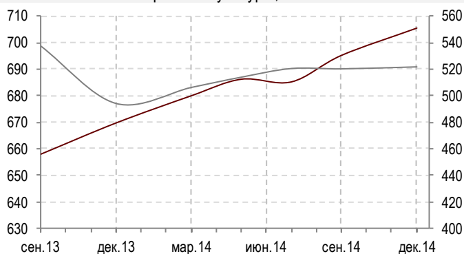
Зерновые культуры, CBOT
