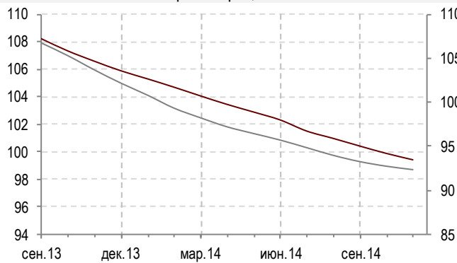
Сырая нефть, NYMEX
